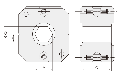
銅線用ダイス寸法図
