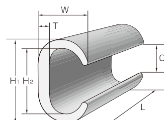
コネクター寸法図
